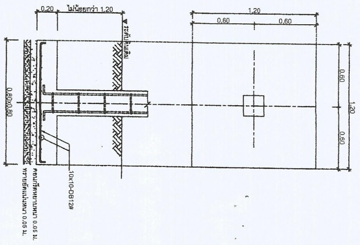
F1 SCALE 1:20
