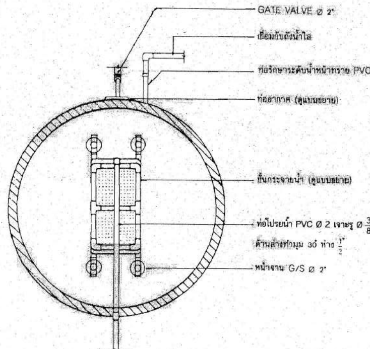
แสดงการวางชั้นกระเจายนํ้าบนถังกรองน้ำ
