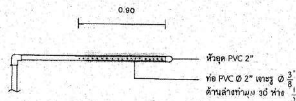
ขนาดท่อโปรยน้ำ
