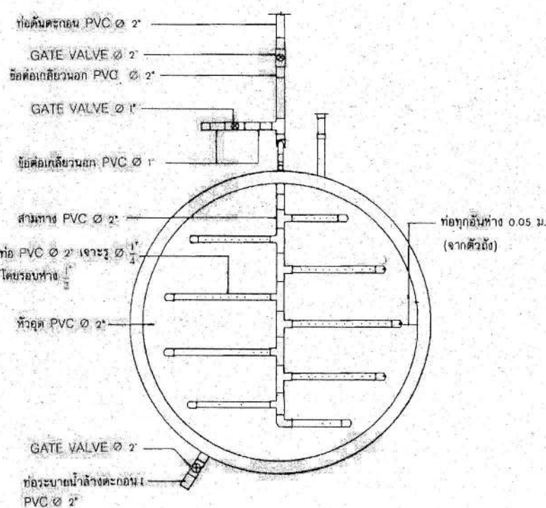
ขยายท่อกรองน้ำ
