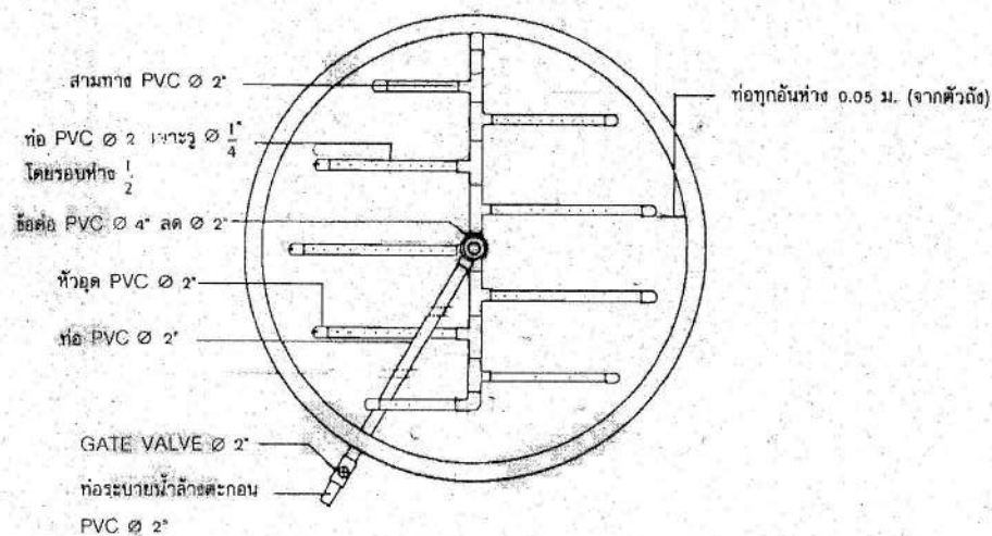
ตำแหน่งกรวยรับน้ำ
