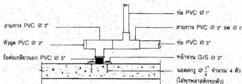
ขยายจุดติดตั้งกระจายน้ำ
