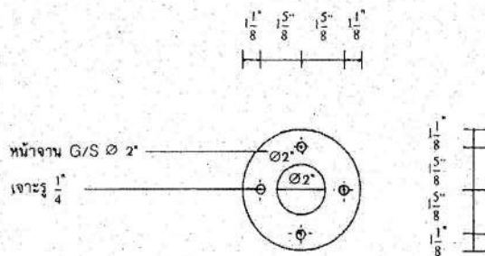
แปลนหน้างาน G/S Ø 2"
