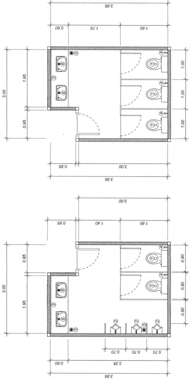
แปลนห้องน้ำชาย
