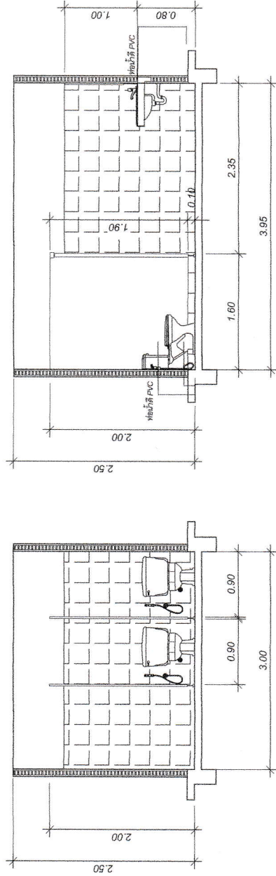
รูปตัดห้องน้ำชาย
